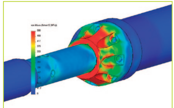
Étude résistance mécanique accouplement
