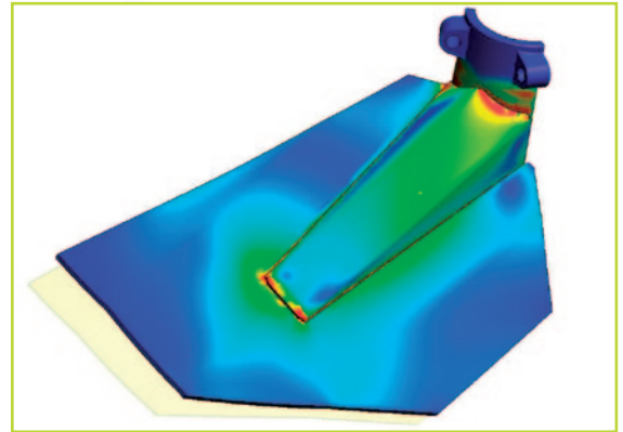
Étude résistance mécanique hélice
